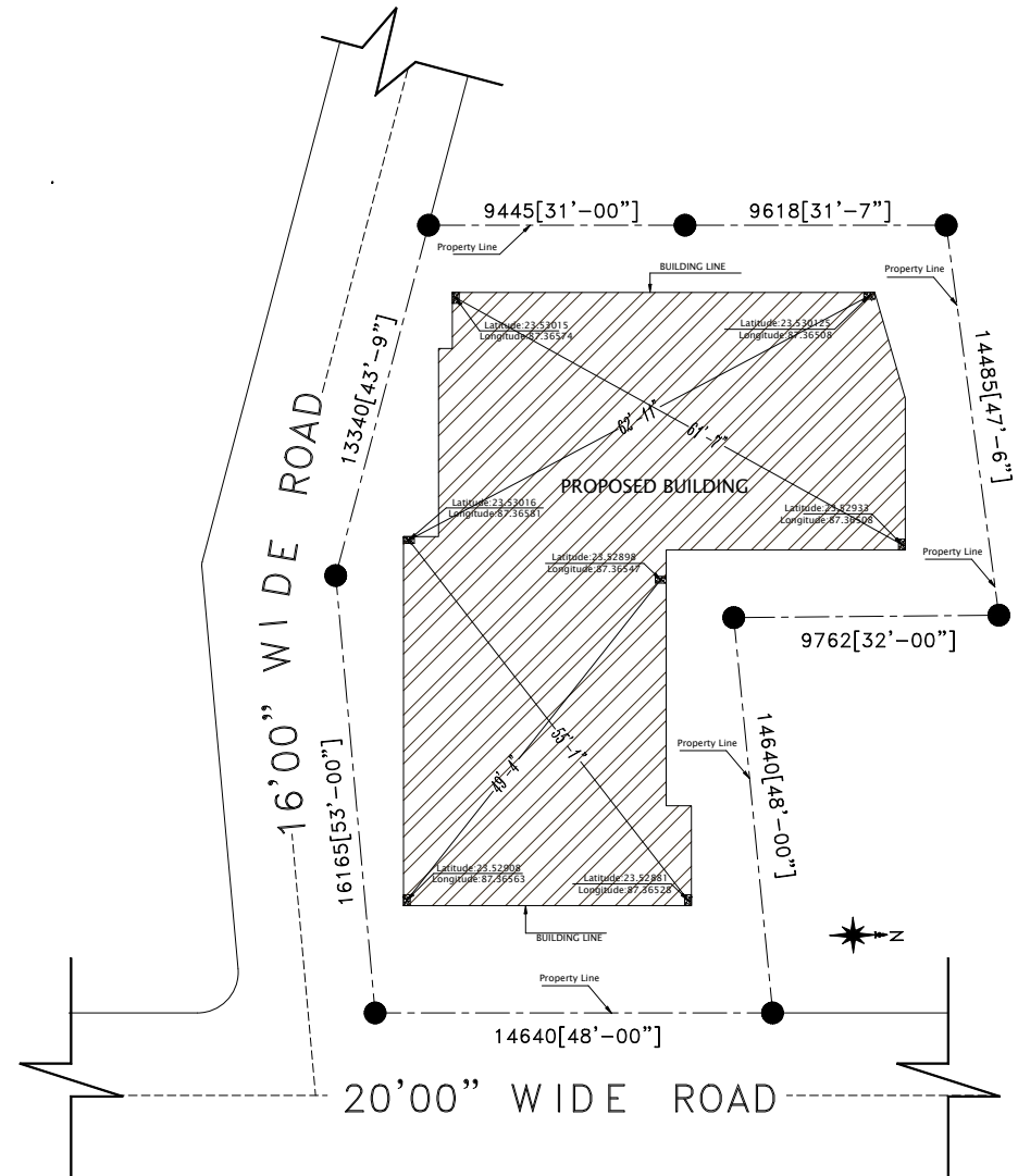
SITE PLAN 1:100
